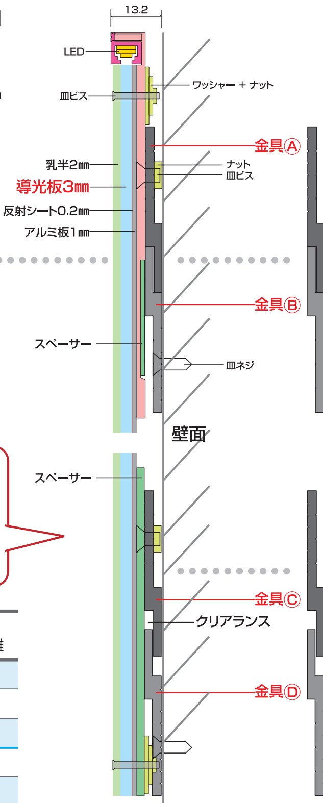
たわみ防止金具を付ける場合の仕様(伸縮対応)
