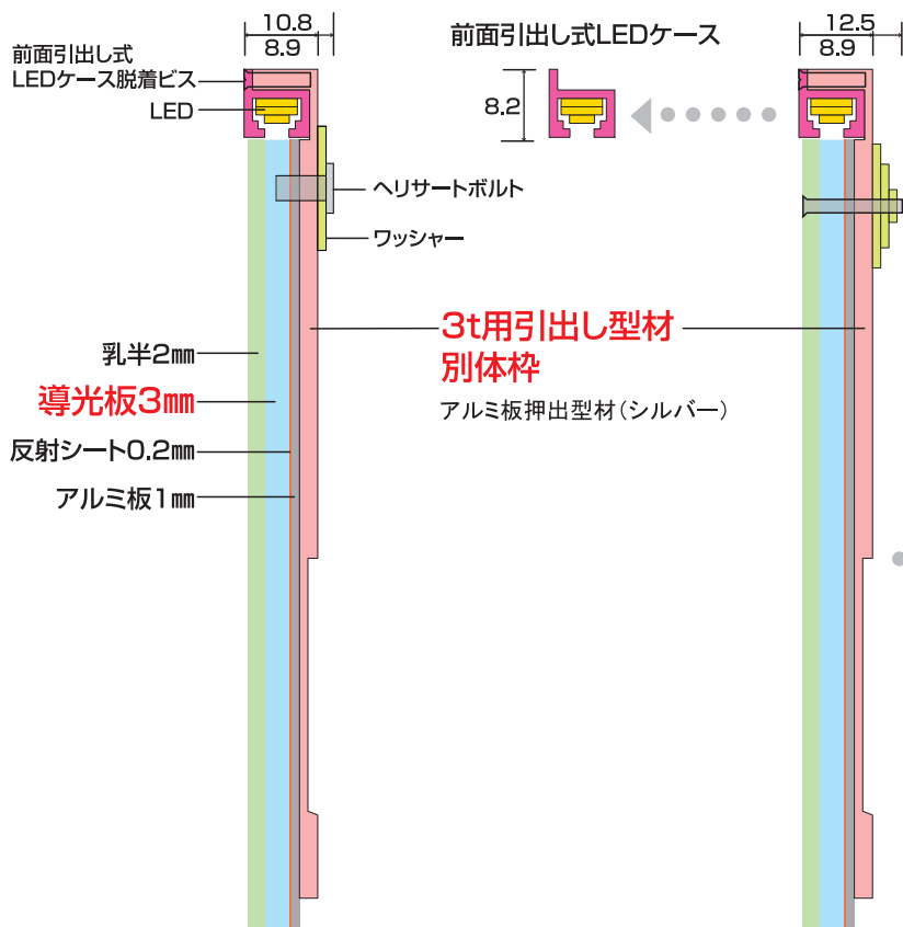
たわみ防止金具を付けない場合の仕様
